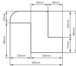
Standard (Bullnose) Z Frame
